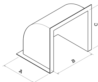
Déflecteurs 600 et 700.
