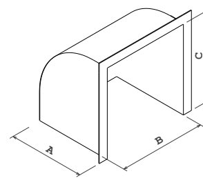
Déflecteurs 500, 950, 1100 et 1400.
